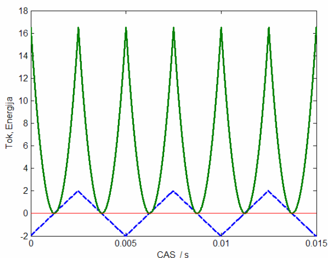
SLIKA: Tok (modra črtkana, v [A]) in skupna energija sistema dveh tuljav (polna črta, v [mJ]). MATLAB: L_{nad}=8.26e-3 ; t=0:1e-6:15e-3 ; \omega=2*\pi/5e-3 ; i=2*sawtooth(\omega.*t,0.5) ; W=1e3*0.5*L_{nad}*i.^2 ; plot(t,i,t,W,t,zeros(1,length(t)))
