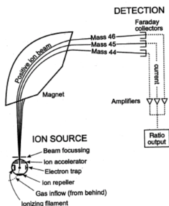
SLIKA: Koncept masnega spektrometra. Vir: Wikipedia.
