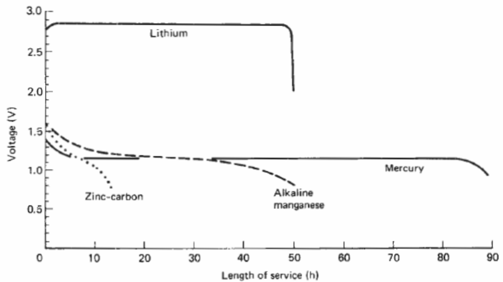
SLIKA: Napetostne karakteristike V(t) različnih tipov baterij. Vir: T.R. Crompton: Battery reference book, Newnes, 2000.
